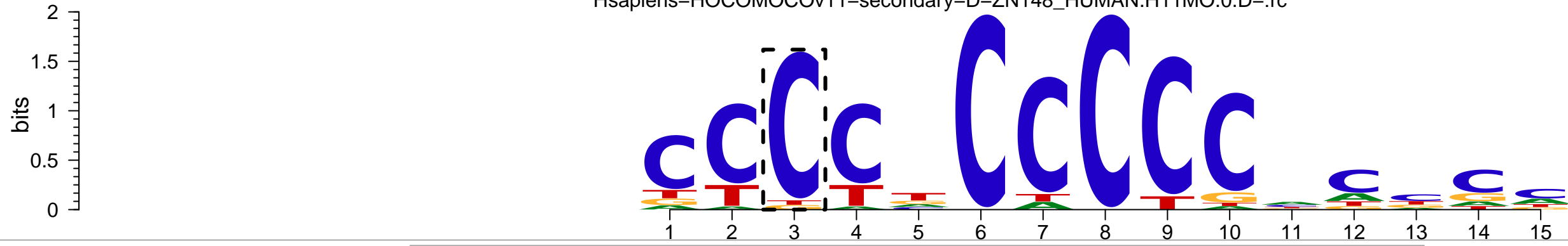
ZN467_motif
