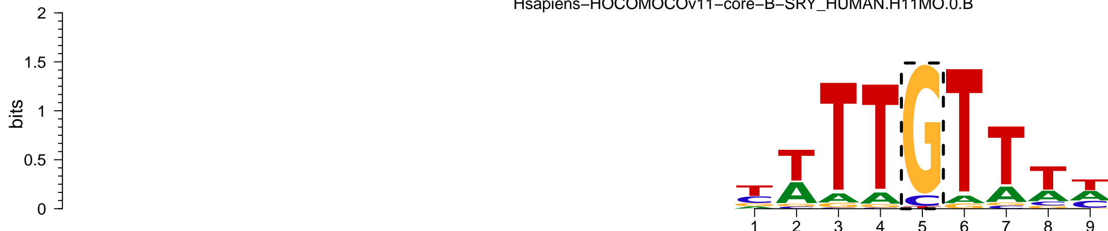
Hsapiens-HOCOMOCov11-core-A-FOXP1_HUMAN.H11MO.0.A
